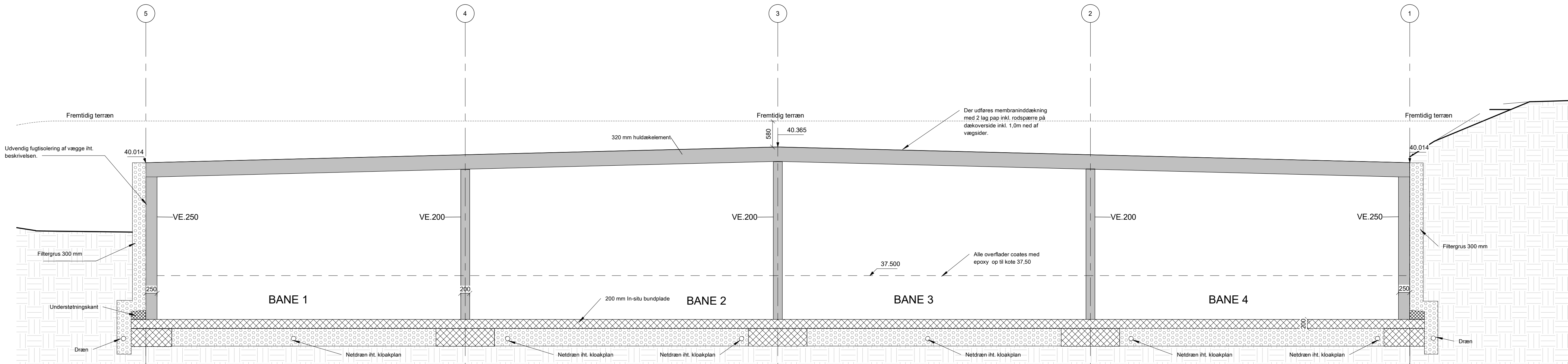
Snit E_E Tværsnit
