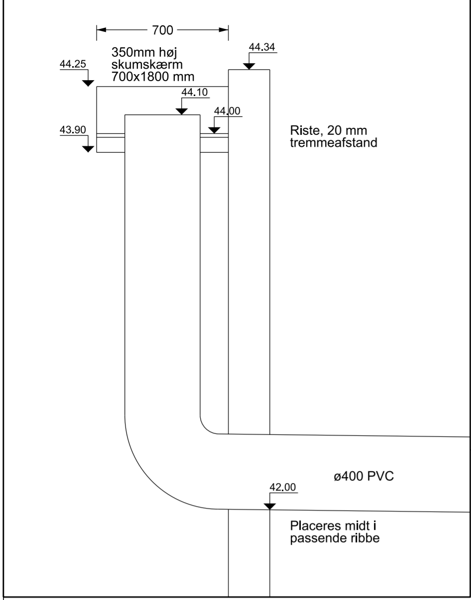
Detail overløb B33270 Mål 1:20
