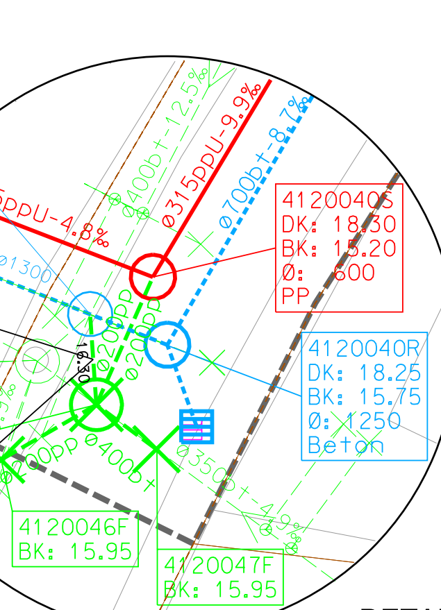
DETALJE Mål 1:200
