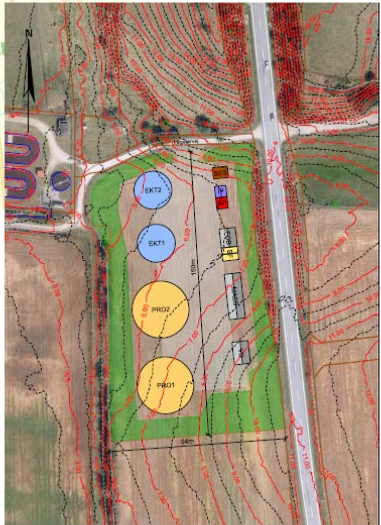
Principskitse for Skals Renseanlæg
